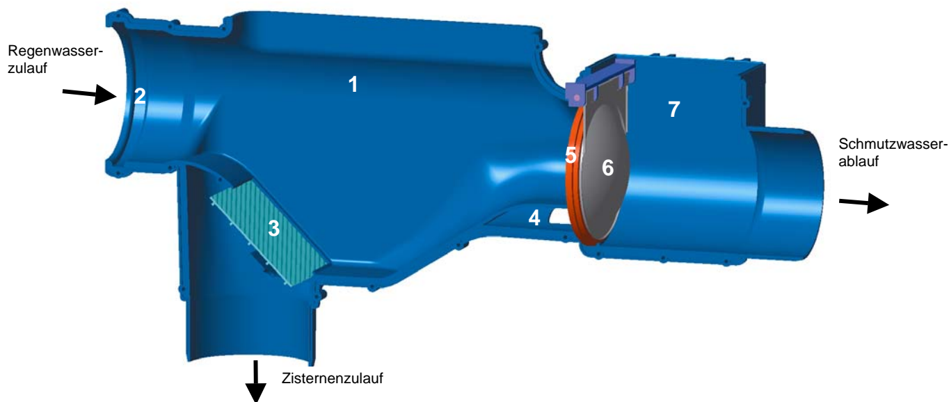
Abb. 1: Aufbau des WSP-Filters
